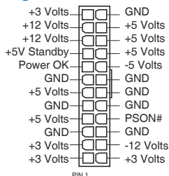
C ATX_PWR
