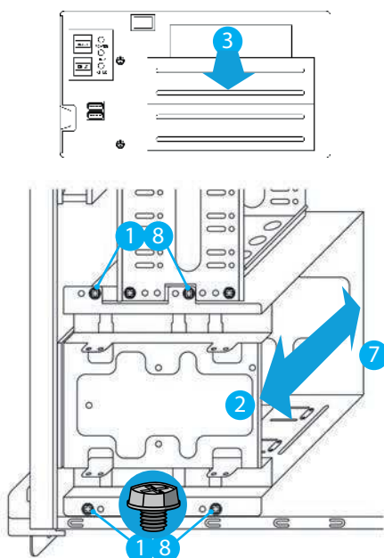
Rysunek 3.4.2.3. Obudowa SC01-4504-10B
