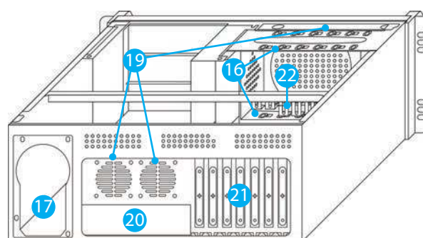
Rysunek 2.6.1.2 - obudowa SC01-4504-08B
