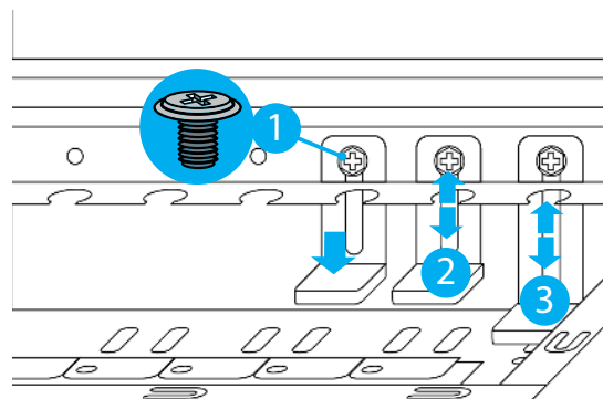
Figure 3.8.1.1. SC01-4504-10B
